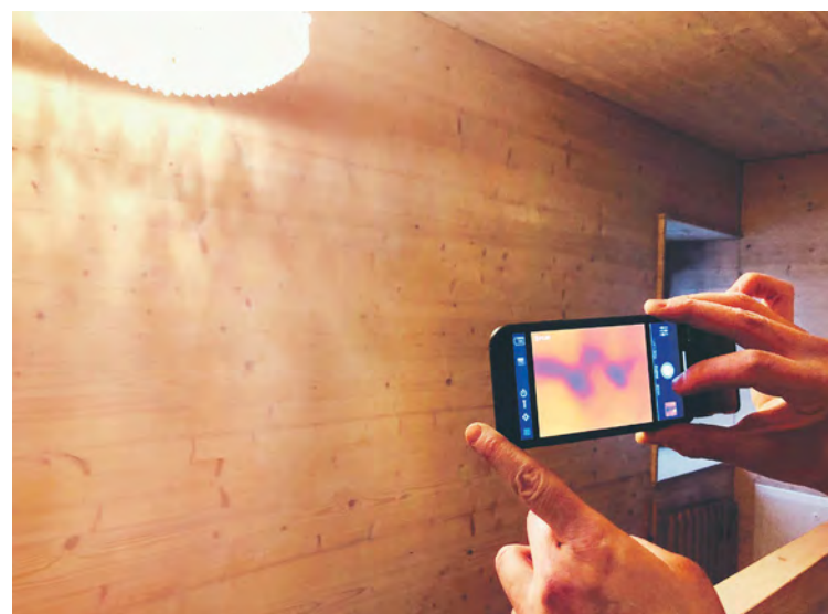
Stora bilden till vänster: De tåliga väggarna gör det enkelt att skapa lekrum med några skruvar och rep. Lilla bilden till höger: Med en enkel värmekamera på mobilen kan man se värmeförluster i väggarna. En elsladd som drar in lite kyla är en köldbrygga. Men viktigare är att hitta de ställen där lite extra isolering stoppar slöseriet.
